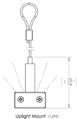
Uplight Mount (UM)
